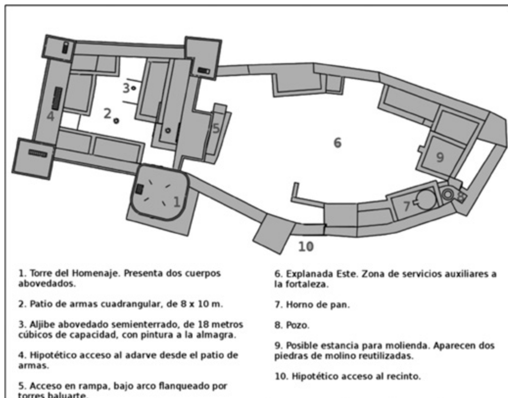
Planta esquemática general de la fortaleza militar y recinto auxiliar. (Fuente: Elaboración propia).
