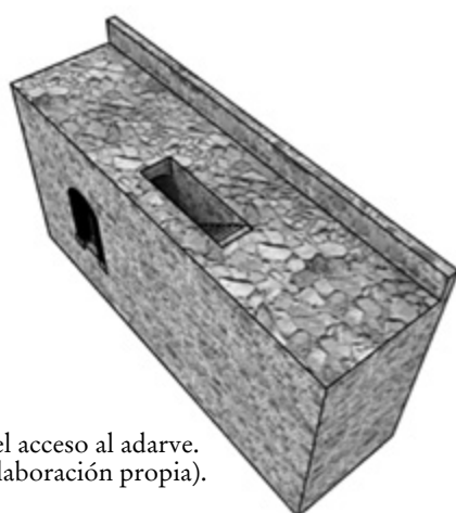
Reconstrucción del lienzo Oeste y acceso al adarve. (Fuente: Elaboración propia).
