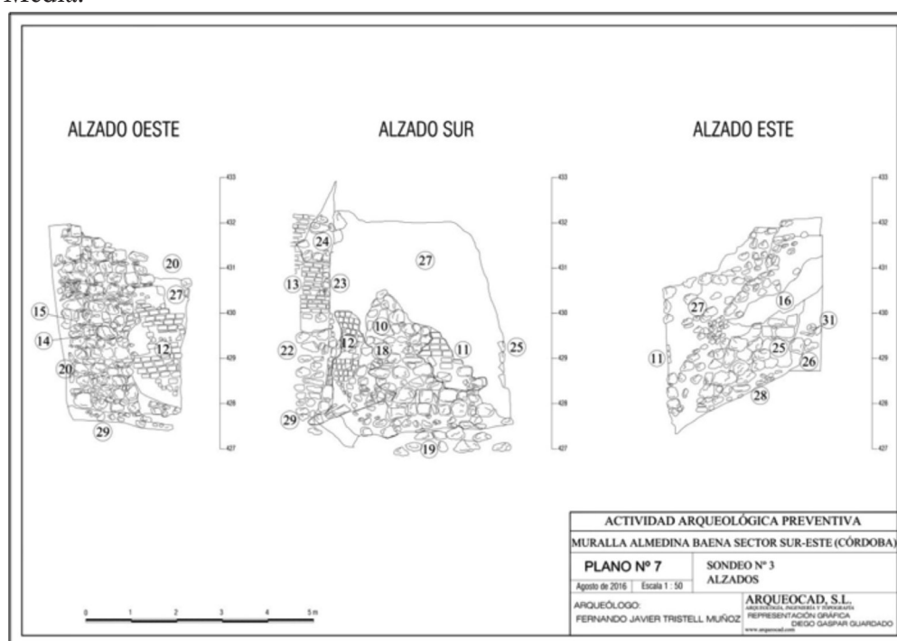
Fase I. Sonda 3. Alzado de los tres flancos de la torre.
