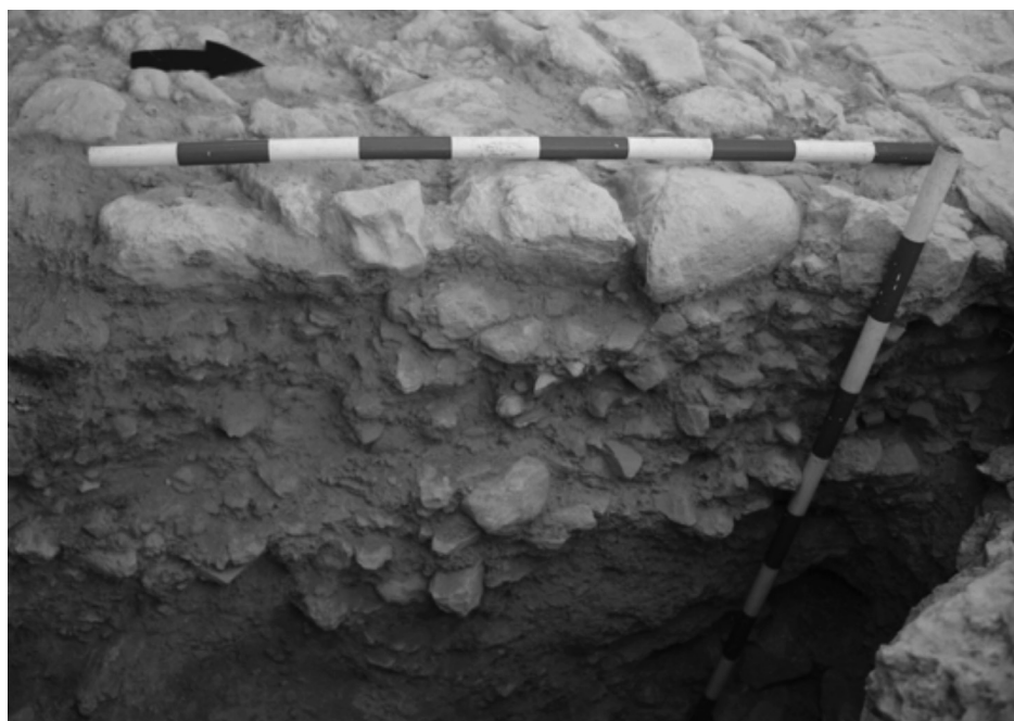
Fase II. Sondeo 2. Vista de las distintas capas del pavimento del andén.
