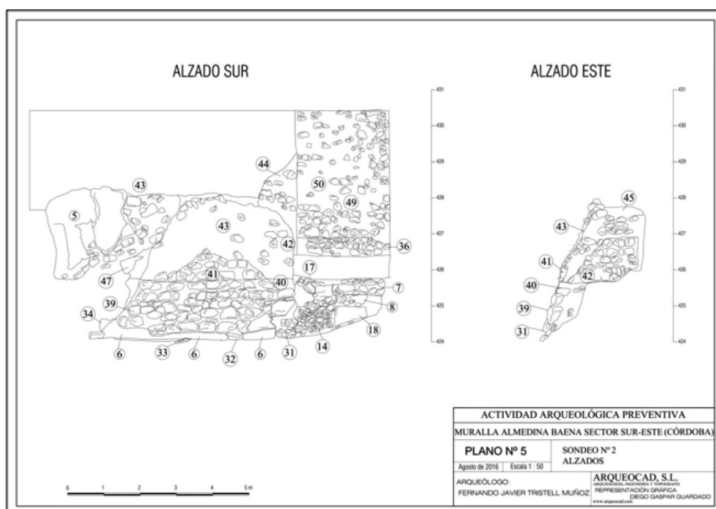
Fase I. Sondeo 2. Alzado de la torre, lienzo de muralla y vivienda adosada.
