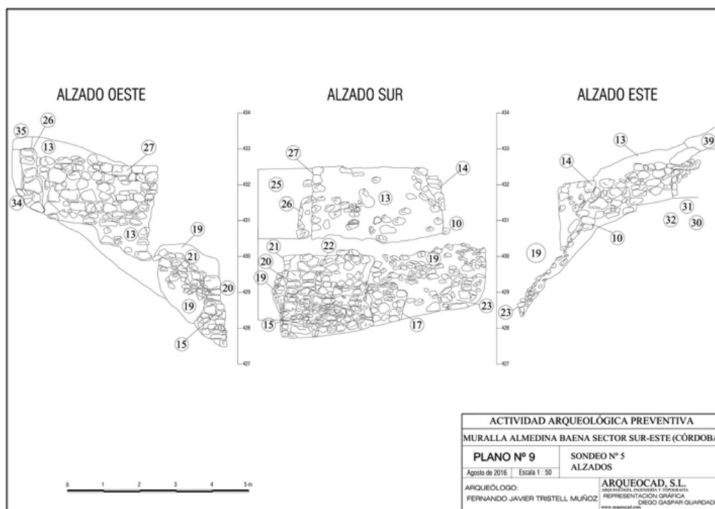
Fase I. Sondeo 5. Alzado de los tres flancos de la torre con zarpa incluida.
